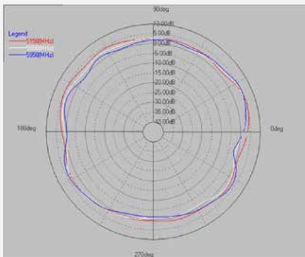
5G (PHI=0)
