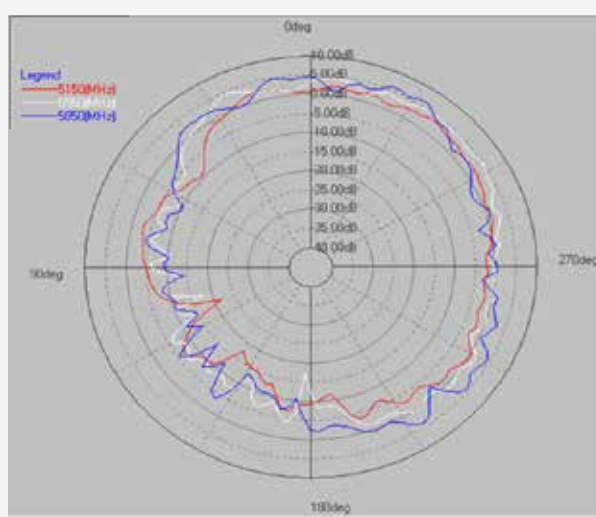
5G (PHI=90)
